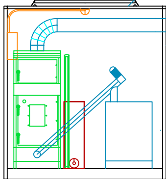
Sez. B-B
